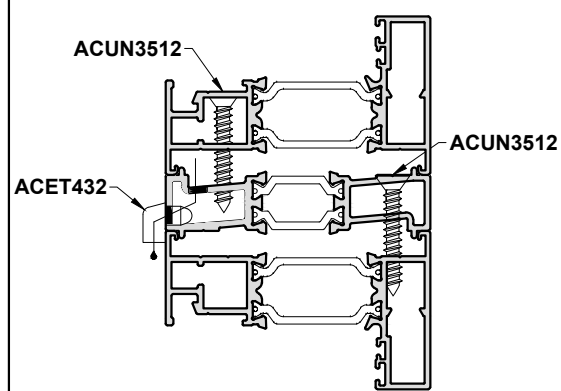
ETC4110
